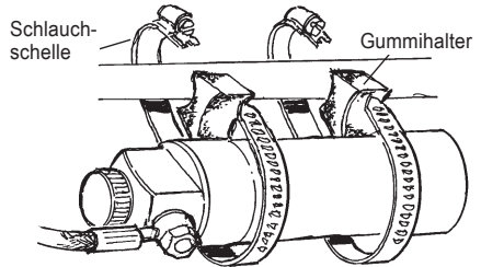
Montage des Reservoirs
